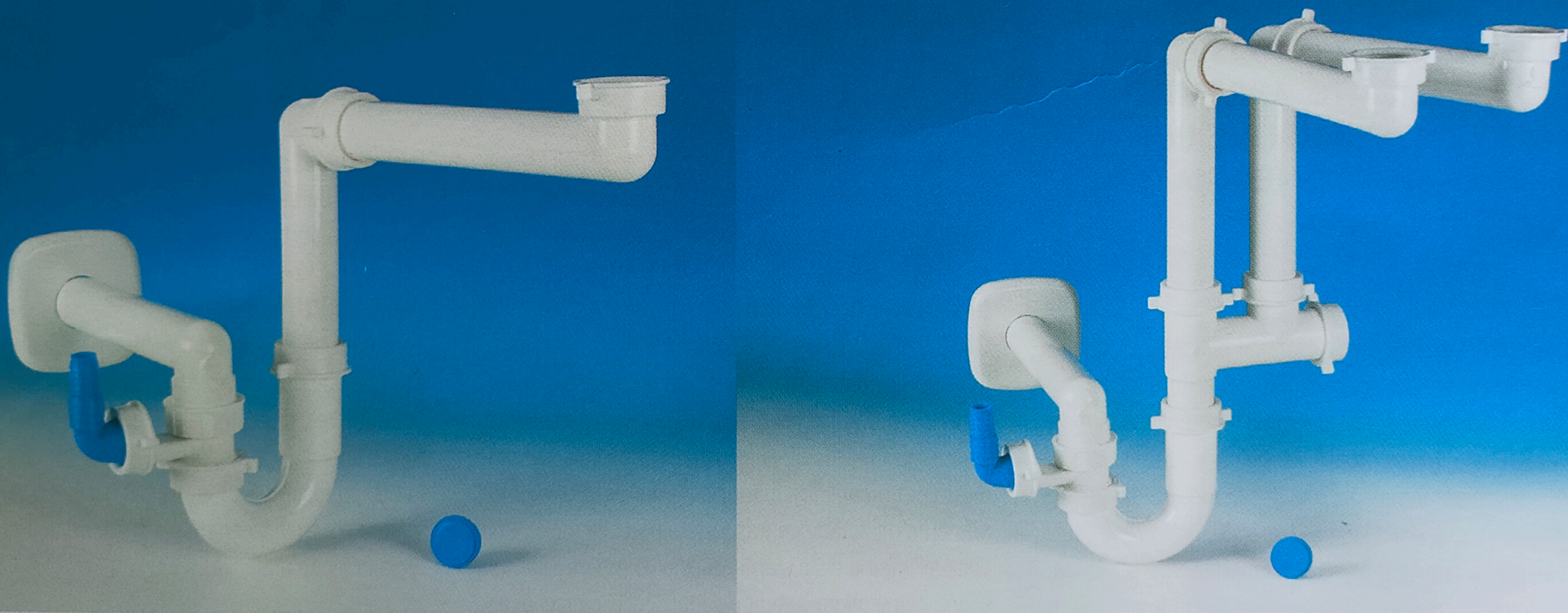
A sinistra: spazio 1 Domestico per lavelli a una vasca. A destra: New Spazio 2 Domestico per lavelli a due vasche
